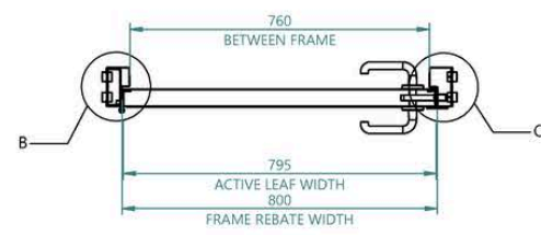
Fig. 6 Section A-A (1:5)
